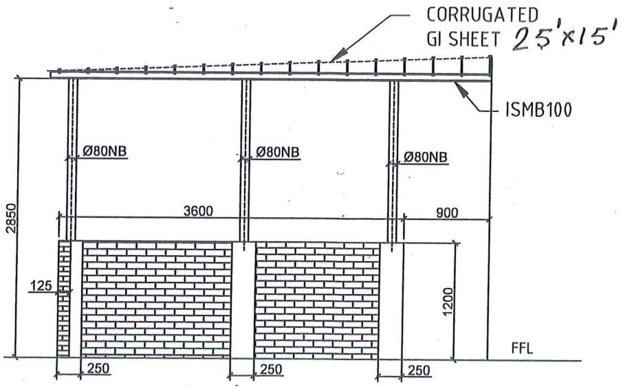
SECTION : X-X
